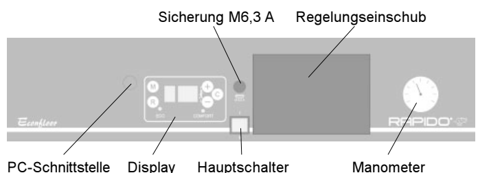
Abb. 4.2 Gesamtansicht des Schaltpultes
