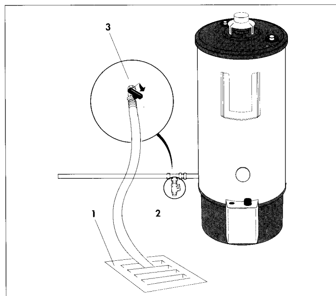
Abb. 6 Entleeren
